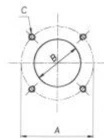
Placa de anclaje
